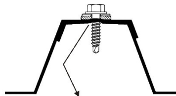
Schraube mit Hinterstich - mit Scheibe -
